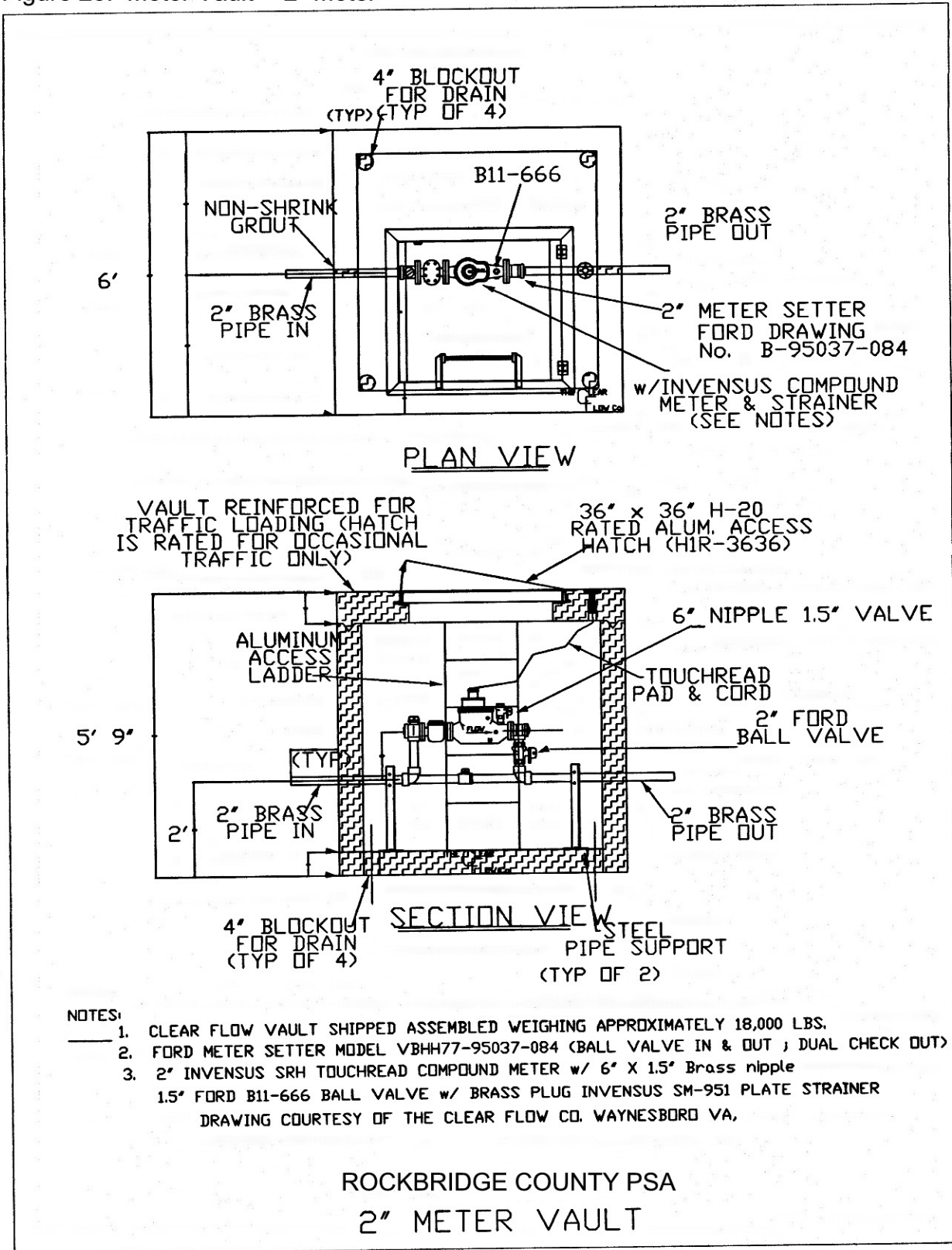
Figure 28. Meter Vault -- 2" Meter
